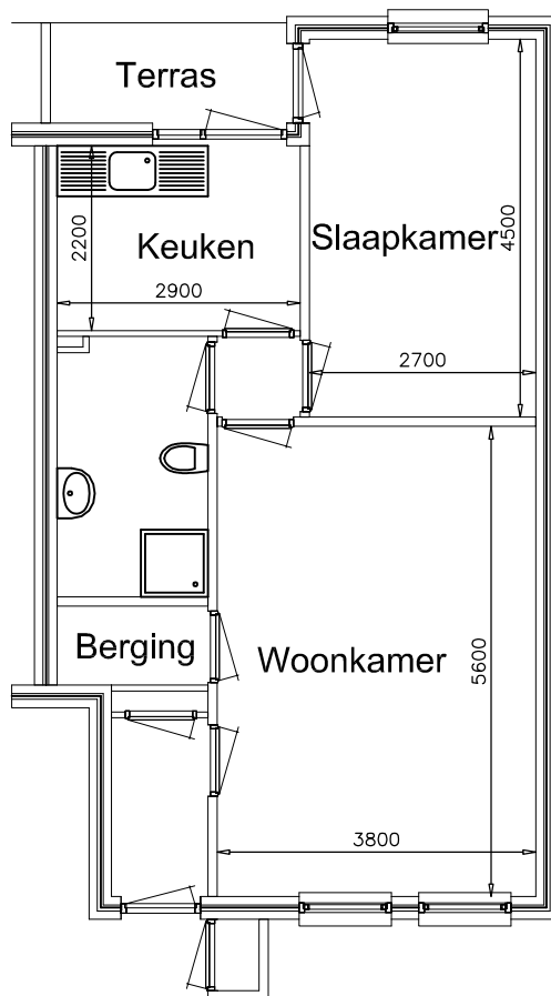
Begane grond
