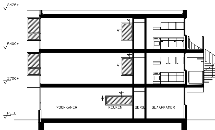
DOORSNEDE
