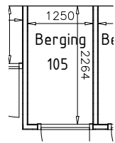
Berging (1e verdieping)
