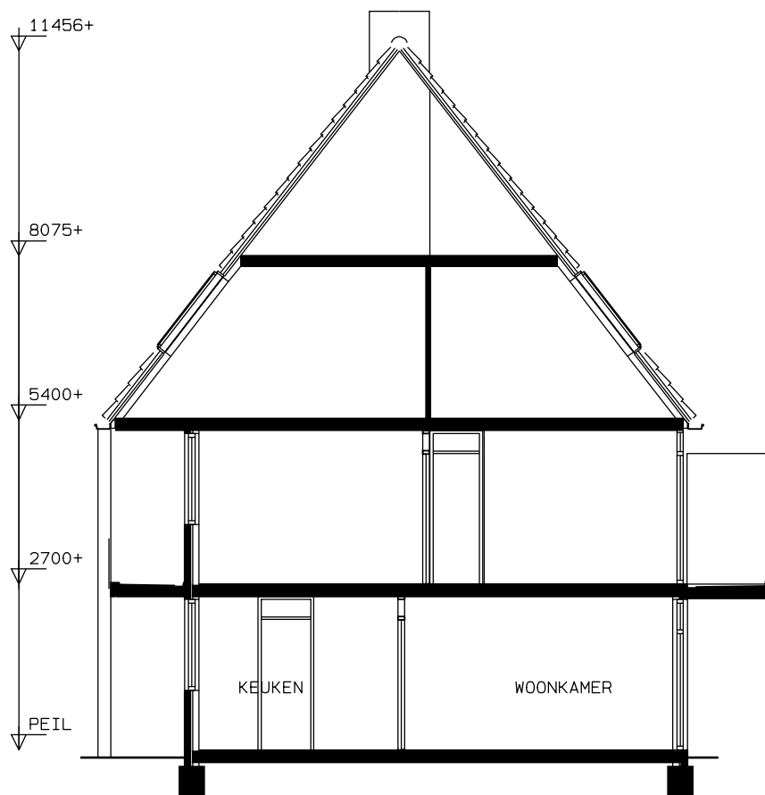
DOORSNEDE
