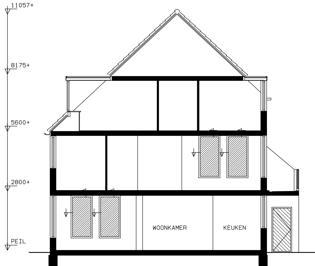
DOORSNEDE
