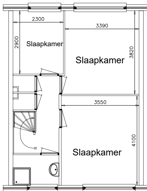
1e verdieping
