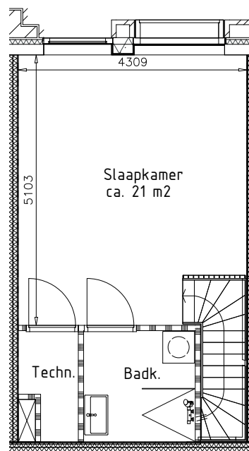
1e verdieping
