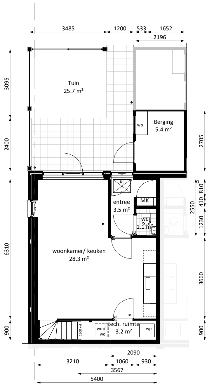
begane grond
