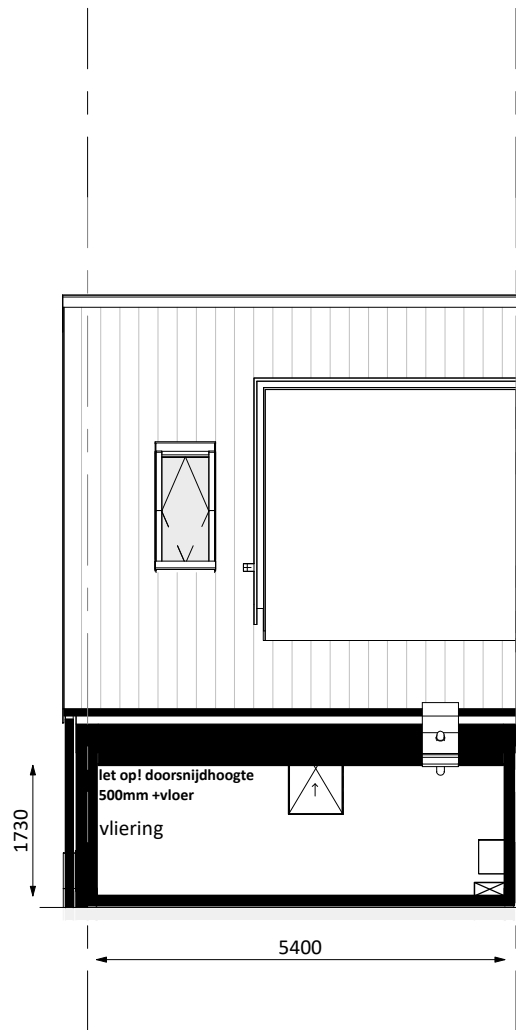
vliering
