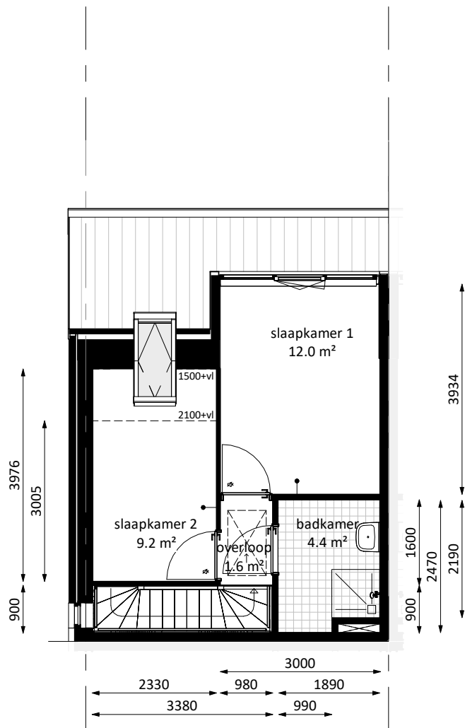
eerste verdieping
