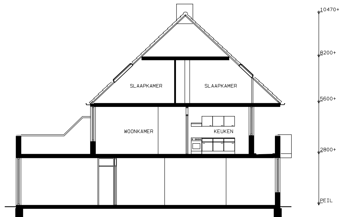
DOORSNEDE
