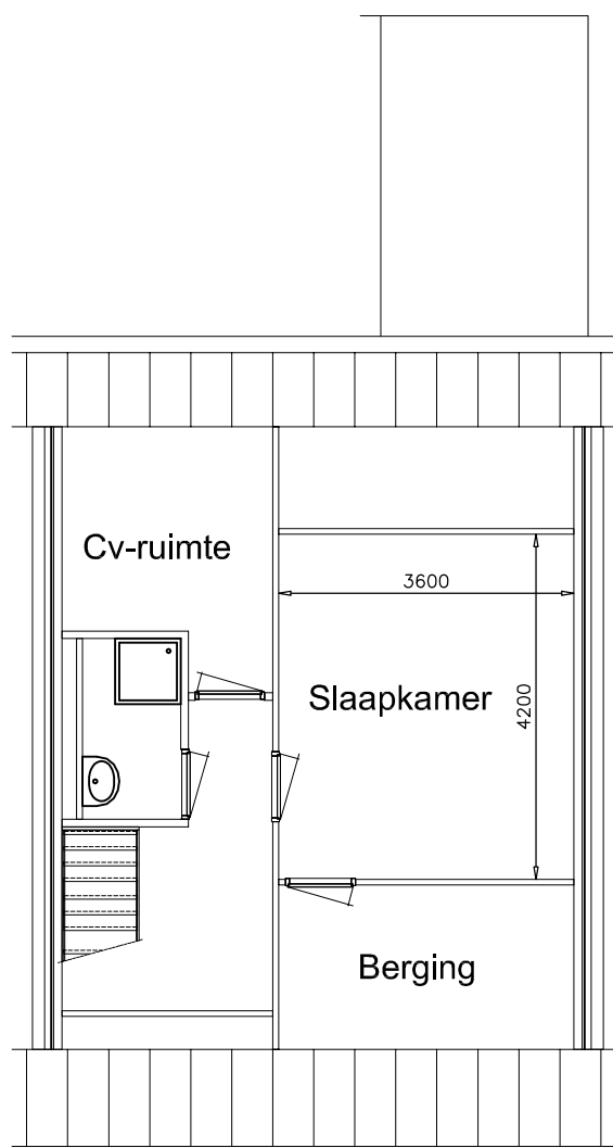
2e verdieping
