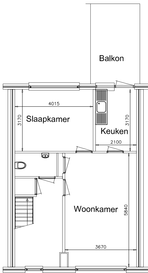
1e verdieping
