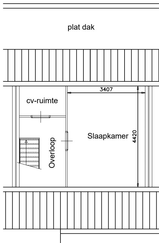
Verdieping
