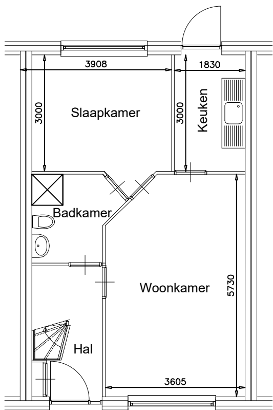
Begane grond
