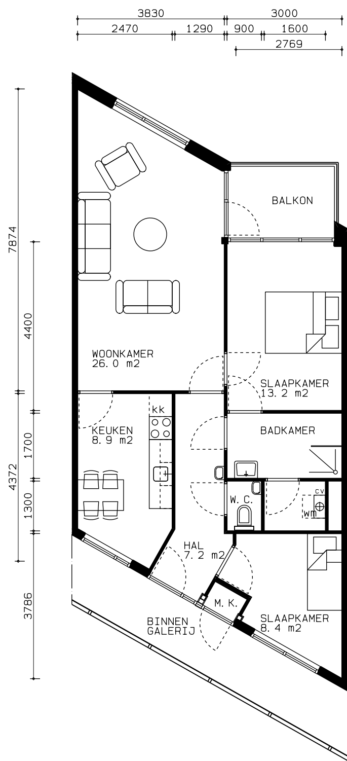
2e VERDIEPING
