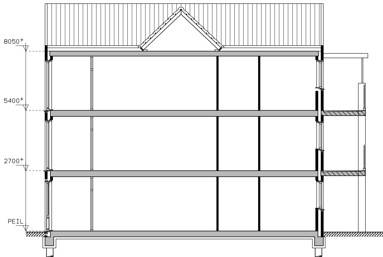
DOORSNEDE
