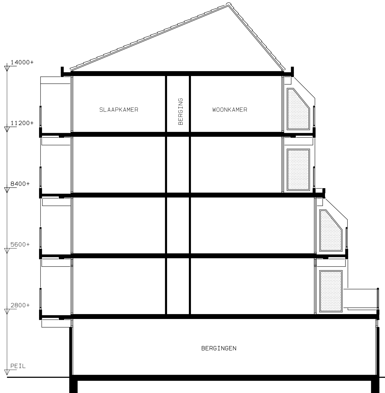
DOORSNEDE
