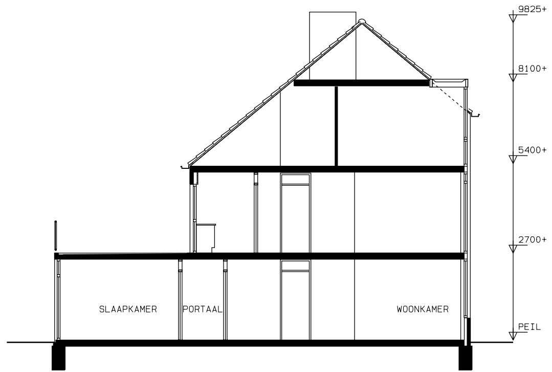
DOORSNEDE
