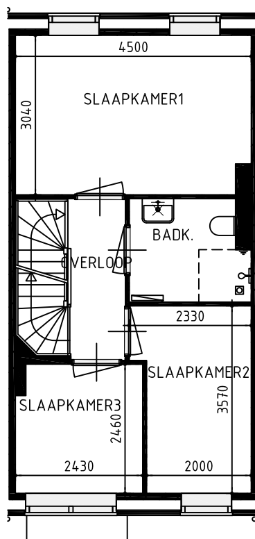
1e verdieping
