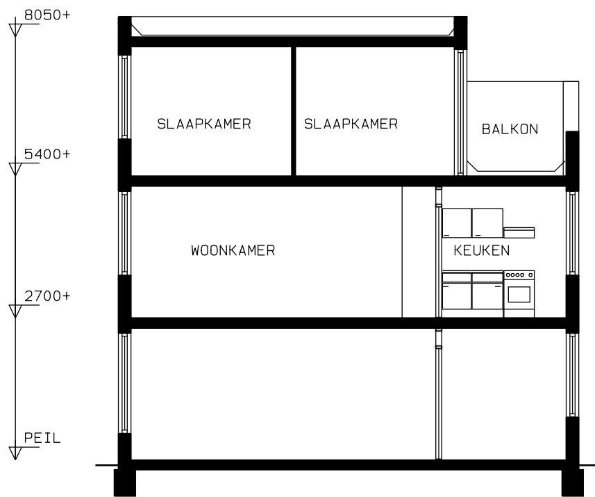
DOORSNEDE
